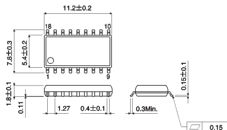
SOP18
